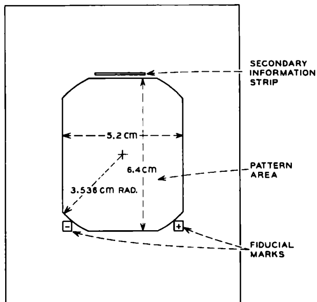
Fig. 3—Reticle format.
