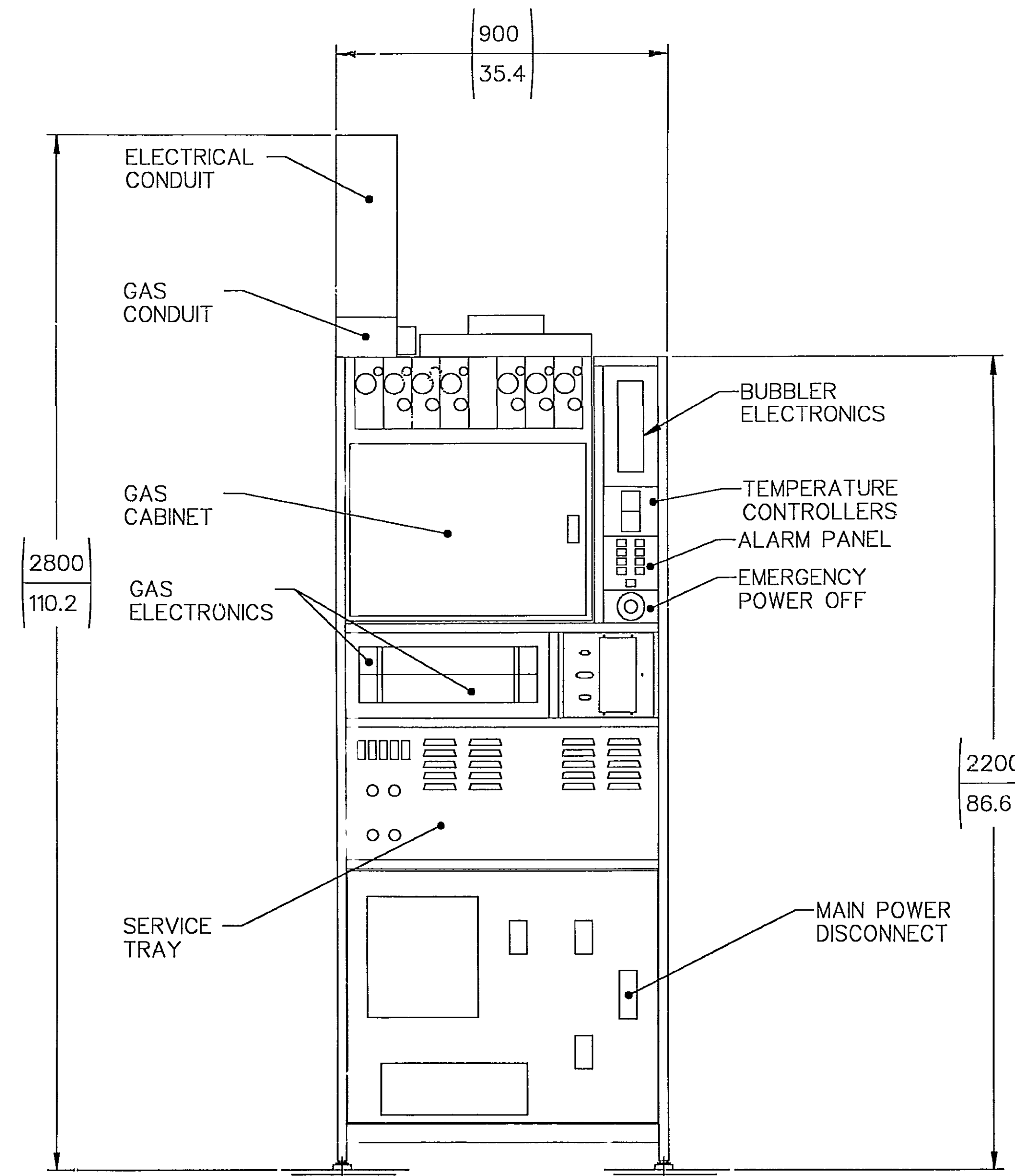
VIEW A-A
