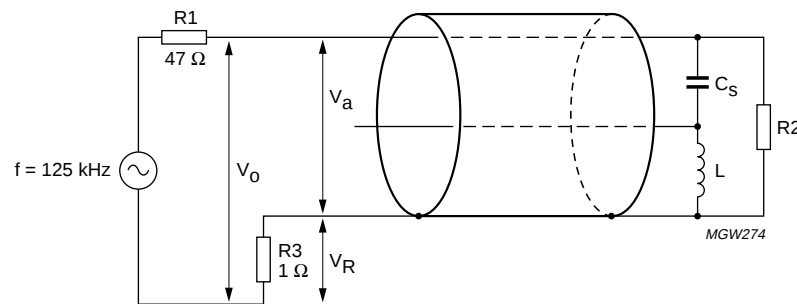
Fig.14 Tuning the antenna.
