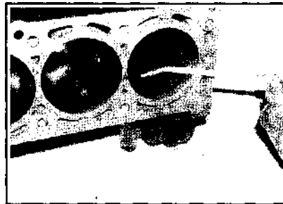
18.9 Смазка поверхности цилиндра перед установкой поршня с шатуном
