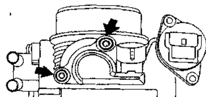
12.21 Винты крепления датчика поворота дроссельной заслонки
