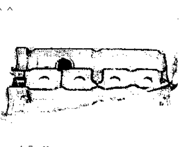
4.7а Уложите прокладку в канавку на крышке головки цилиндров...
