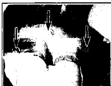
15.1a Болты крепления передней выхлопной трубы (стрелки)
