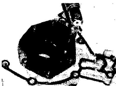
14.7а Отверните винты и снимите крышку насоса
