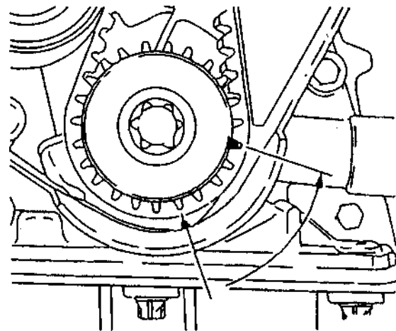
11.3 Перед снятием ремня проверните выставьте поршень 1-го цилиндра в ВМТ такта сжатия и поверните коленвал назад на 60°
