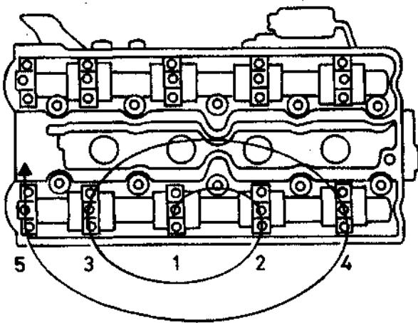
10.12в Спиральный порядок затягивания болтов крышек распределов
