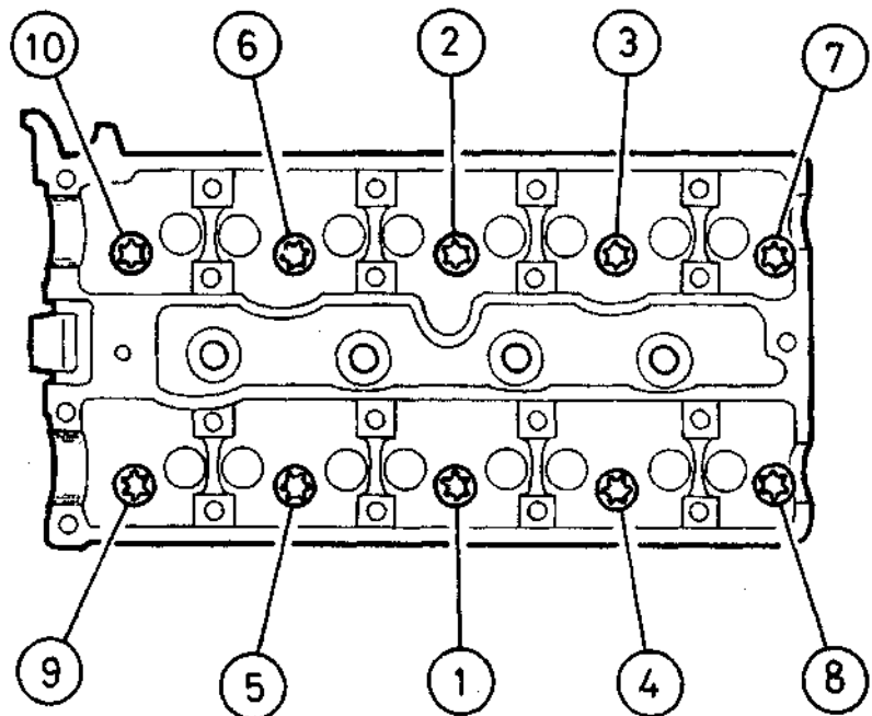
11.30а Последовательность затяжки болтов головки цилиндров (все Двухвальные двигатели)
