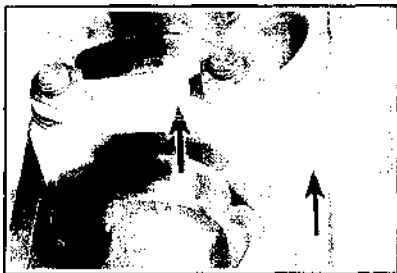
10.3б Место нанесения номеров на крышках опорных шеек распредвала и на постелях головки цилиндров
