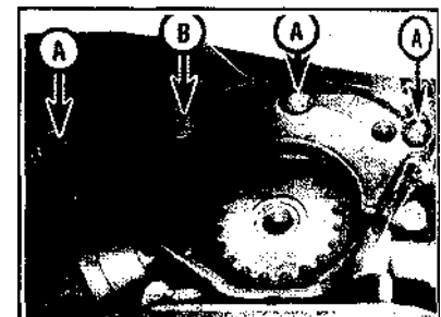
6.6 Болты крепления нижней крышки (А) и болт натяжителя ремня распределителя (В)
