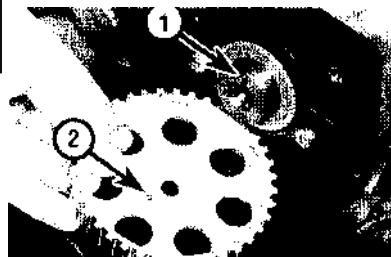
8.3а Установите звездочку по месту так, чтобы штифт на торце распредвала (1) зашел в отверстие на звездочке (2)
