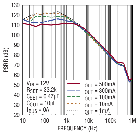
PSRR vs I OUT
